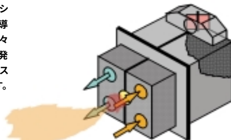
蓄熱燃焼バーナー
