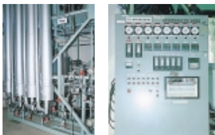
小型試験装置（能力：200リットル/日）
